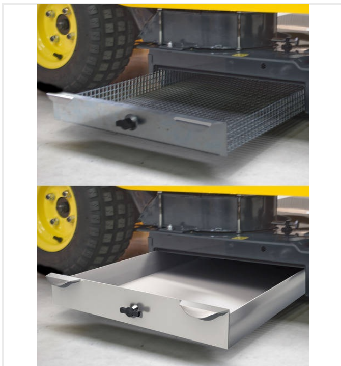
Bandeja de residuos regulable, de 4 - 10 mm
